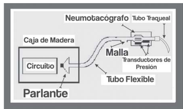
Fig. 3. Esquema del sistema para medir FOT.
